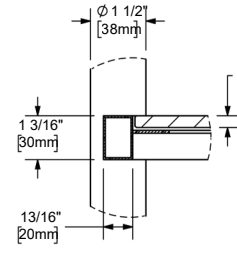
DETAIL BV 1 : 4
