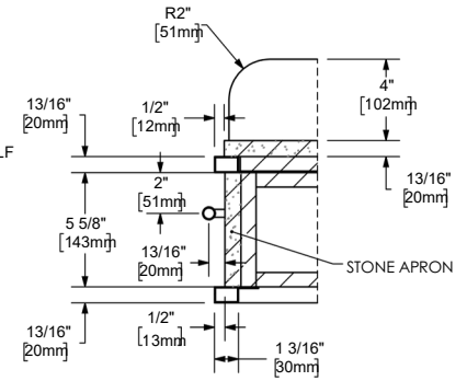
DETAIL BU 1 : 8
